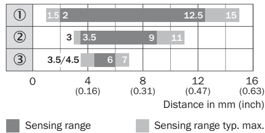
Figura 2: Distância de comutação 15 mm
