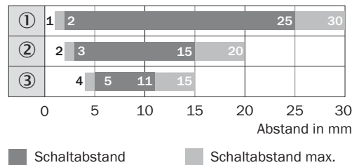
Abbildung 3: Schaltabstand 30 mm
