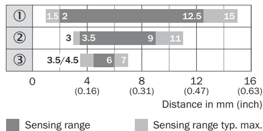
插图 2: 触发感应距离 15 mm
