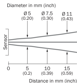
插图 4: GTE2F, 15 毫米版本
