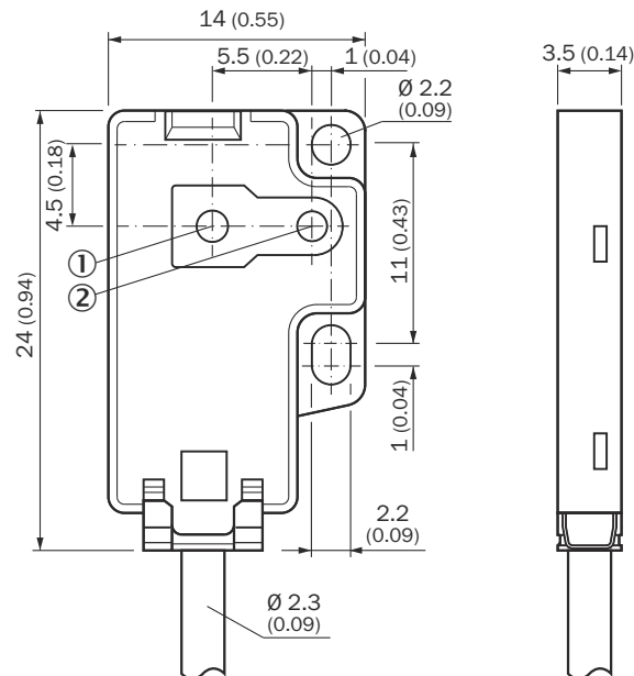
Rysunek 6: Rysunek wymiarowy GTE2F
