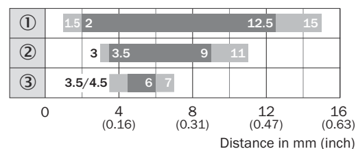
Rysunek 4: Zasięg 15 mm
