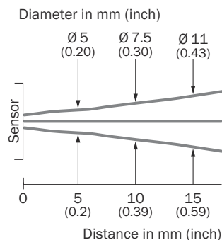
Figura 4: GTE2F, versión de 15 mm
