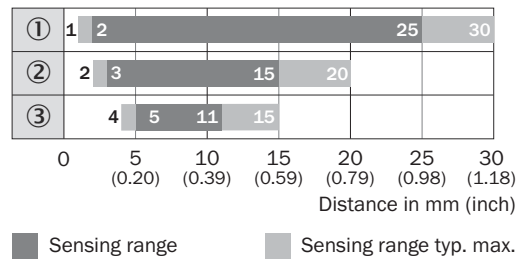
Rysunek 5: Zasięg 30 mm
