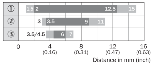
図 2: 検出距離 15 mm
