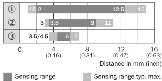
Figura 2: Distancia de conmutación 15 mm
