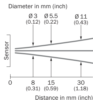
Figura 5: GTE2F, versione da 30 mm
