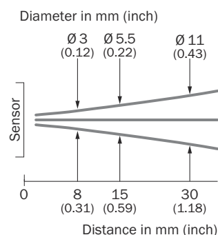
插图 5: GTE2F, 30 毫米版本
