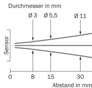
Abbildung 5: GTE2F, 30 mm version
