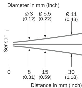
Rysunek 8: GTE2F, wersja 30 mm
