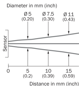
図 4: GTE2F, 15 mm 版
