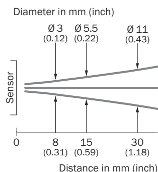
図 5: GTE2F, 30 mm 版
