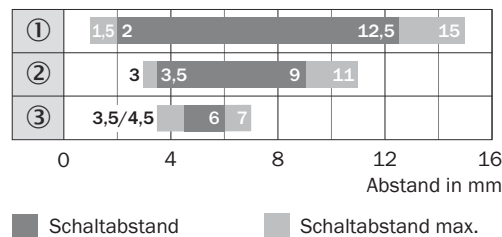
Abbildung 2: Schaltabstand 15 mm
