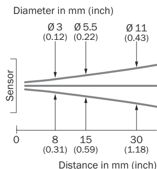
Figura 5: GTE2F, 30 mm version
