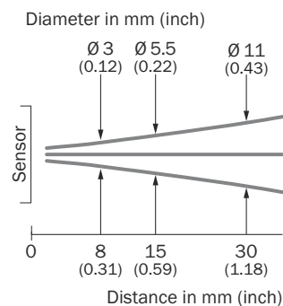
Figura 5: GTE2F, versão 30 mm
