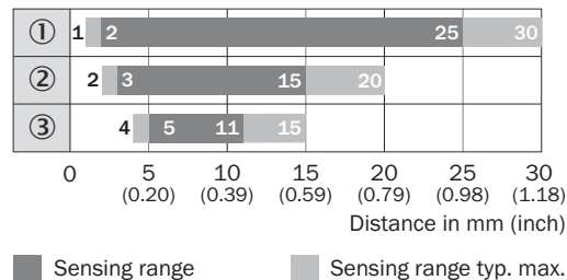
Рисунок 3: Расстояния срабатывания 30 мм
