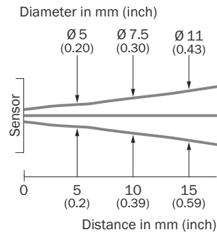
Rysunek 7: GTE2F, wersja 15 mm
