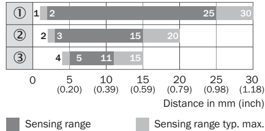
Figura 3: Distância de comutação 30 mm
