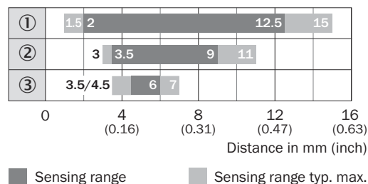
Рисунок 2: Расстояния срабатывания 15 мм
