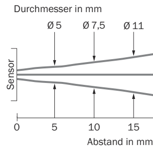
Abbildung 4: GTE2F, 15 mm version
