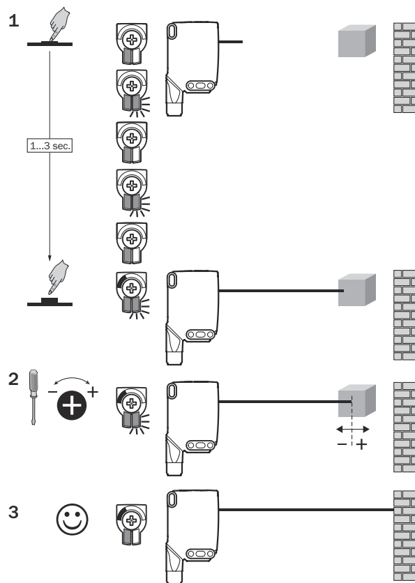
Figura 32: WTB26x-xxxxx2xAxx, ajuste de la distancia de conmutación con un elemento de presión y rotación
