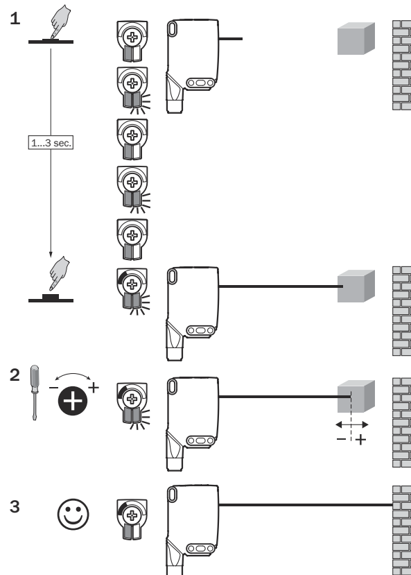
Rysunek 80: WTB26x-xxxxx2xAxx, ustawianie zasięgu za pomocą elementu przyciskowo-obrotowego
