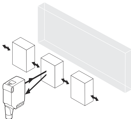
図 61: 対象物に対するセンサの相対的な方向
