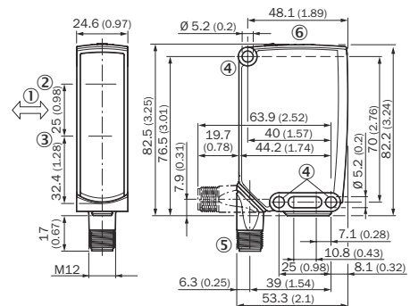
Figura 96: Desenho dimensional 2, conector macho
