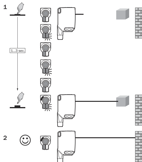
插图 118: WTB26x-xxxxxx3xAxx, 通过示教键调整触发感应距离
