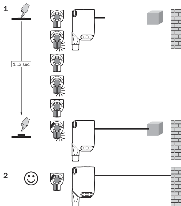
図 70: WTB26x-xxxxxx3xAxx, ティーチンボタンによる検出距離の設定
