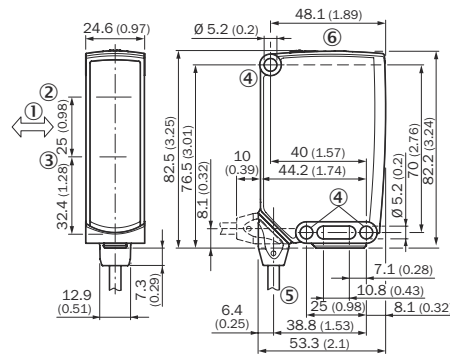
図 71: 寸法図 1、ケーブル
