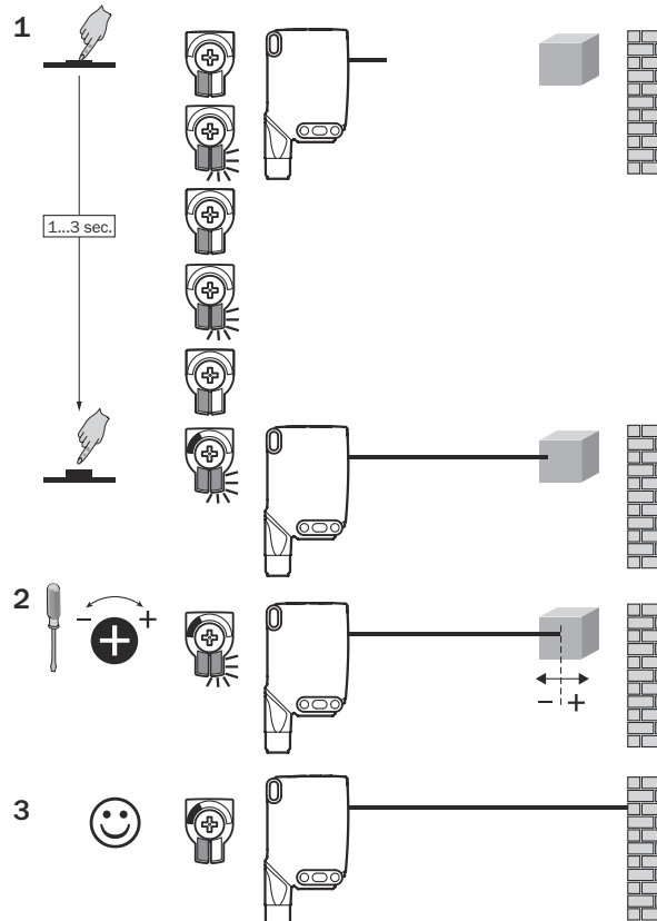
Figura 92: WTB26x-xxxxx2xAxx, ajuste da distância de comutação com elemento de pressão e giro
