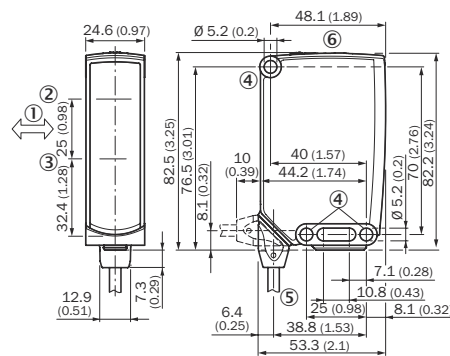
插图 119: 尺寸图 1, 电缆
