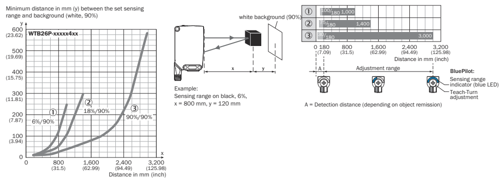
插图 113: 特征曲线 2, WTB26P-xxxx4xx, 红光
