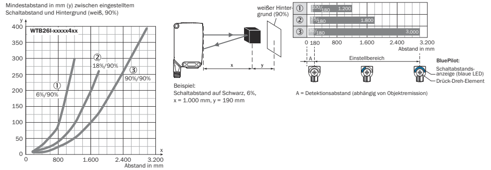
Abbildung 7: Kennlinie 4, WTB26l-xxxxx4xx, Infrarotlicht
