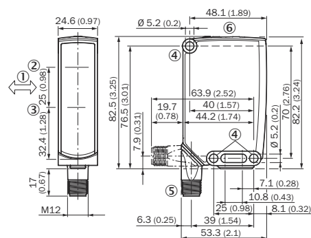
Рисунок 108: Масштабный чертёж 2, штекер
