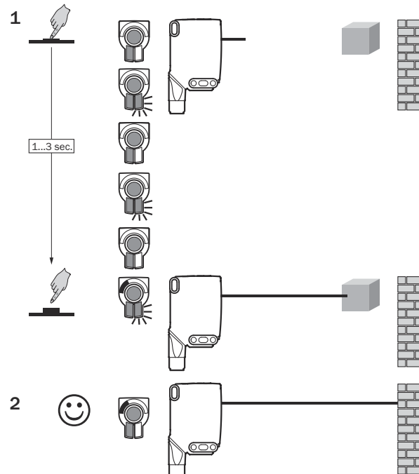
Figura 34: WTB26x-xxxxx3xAxx, ajuste de la distancia de conmutación con una tecla teach-in
