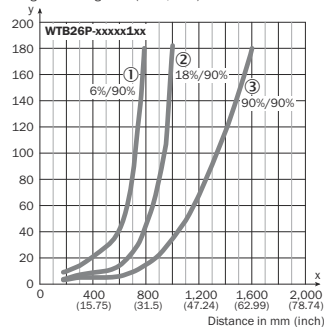
Figura 52: Linea caratteristica 1, WTB26P-xxxxx1xx, luce rossa
