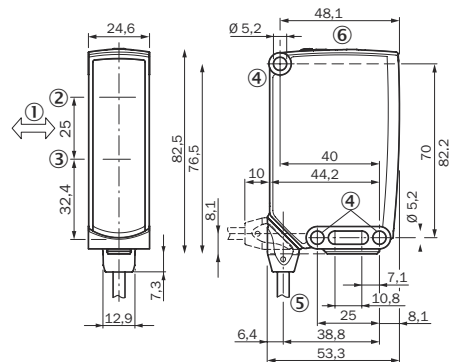
Abbildung 11: Maßzeichnung 1, Leitung
