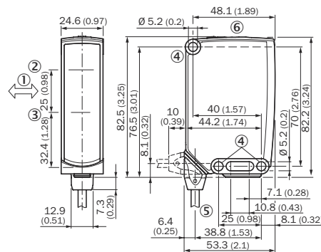
Figura 95: Desenho dimensional 1, cabo
