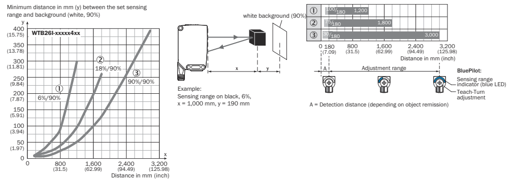
插图 115: 特征曲线 4, WTB26l-xxxxx4xx, 红外光
