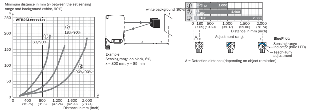
図 66: 特性曲線 3, WTB26I-xxxxx1xx, 赤外光
