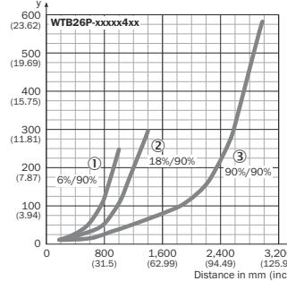
Рисунок 101: Характеристика 2, WTB26P-xxxxx4xx, красный свет
