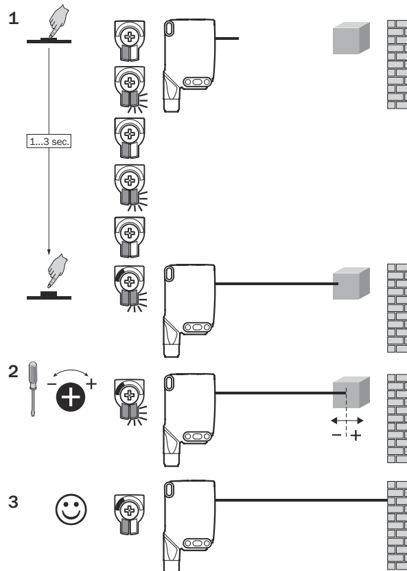
Abbildung 8: WTB26x-xxxxx2xAxx, Einstellung des Schaltabstands mit Drück-Dreh-Element
