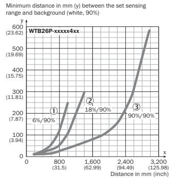
Illustration 41: Caractéristique 2, WTB26P-xxxxx4xx, lumière rouge
