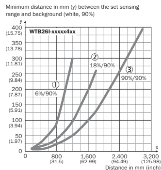
Illustration 43: Caractéristique 4, WTB26I-xxxxx4xx, lumière infrarouge
