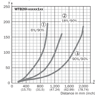
Рисунок 102: Характеристика 3, WTB26I-xxxxx1xx, инфракрасный свет
