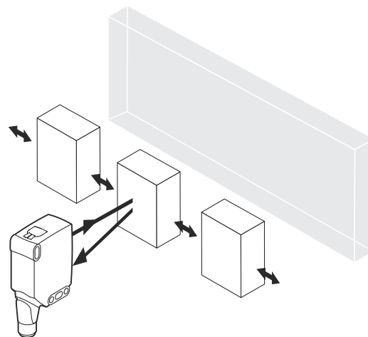
Figura 25: Orientación del sensor respecto a la dirección del objeto
