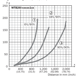
Figura 30: Curva característica 3, WTB26I-xxxx1xx, luz infrarroja
