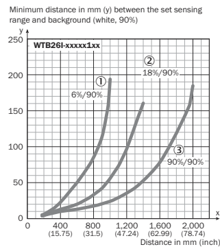
Illustration 42: Caractéristique 3, WTB26I-xxxxx1xx, lumière infrarouge
