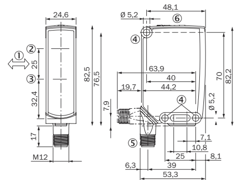
Abbildung 12: Maßzeichnung 2, Stecker
