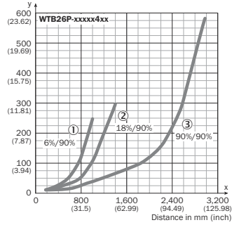
Figura 29: Curva característica 2, WTB26P-xxxx4xx, luz roja
