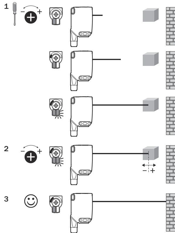
Figura 33: WTB26x-xxxxx1xAxx, ajuste de la distancia de conmutación con un potenciómetro
