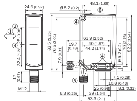
Figura 36: Dibujo acotado 2, conector macho
