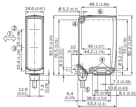
Rysunek 83: Rysunek wymiarowy 1, przewód
