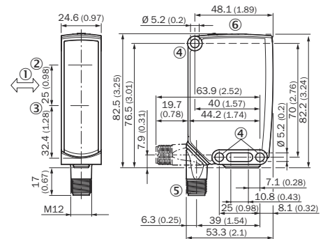
図 72: 寸法図 2、オスコネクタ
