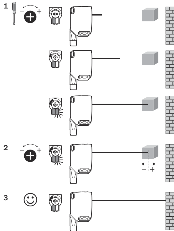
Rysunek 81: WTB26x-xxxxxx1xAxx, ustawianie zasięgu za pomocą potencjometru
