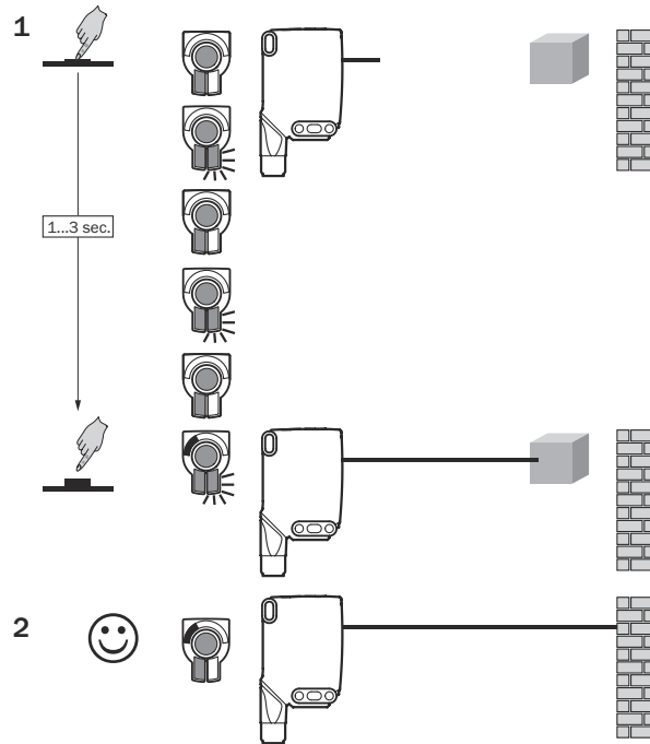
Abbildung 10: WTB26x-xxxxx3xAxx, Einstellung des Schaltabstands mit Teach-in-Taste
