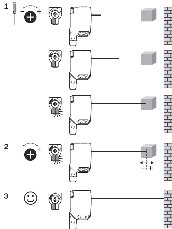
插图 117: WTB26x-xxxxxx1xAxx, 通过电位计调整触发感应距离
