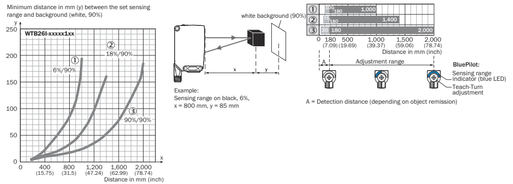
Figura 90: Curva característica 3, WTB26I-xxxxx1xx, luz vermelha
