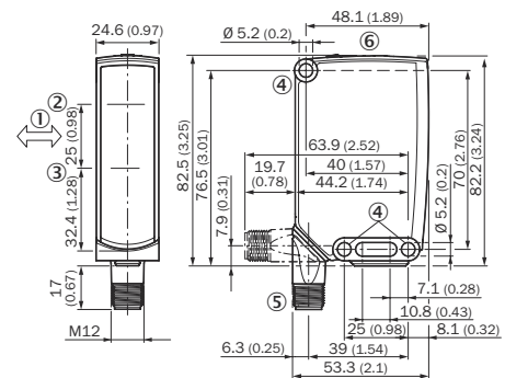
插图 120: 尺寸图 2, 插头
