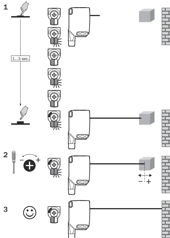
Figura 56: WTB26x-xxxxx2xAxx, impostazione della distanza di lavoro con regolazione a pressione rotazione
