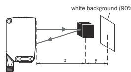
Рисунок 101: Характеристика 2, WTB26P-xxxxx4xx, красный свет
