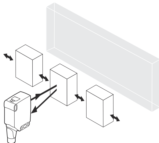
Рисунок 97: Ориентация датчика по отношению к направлению объекта
