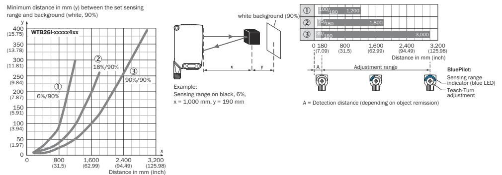
図 67: 特性曲線 4, WTB26I-xxxxx4xx, 赤外光
