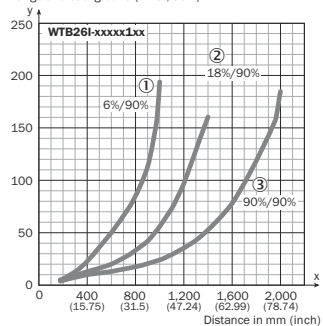
Rysunek 78: Charakterystyka 3, WTB26I-xxxx1xx, światło podczerwone
