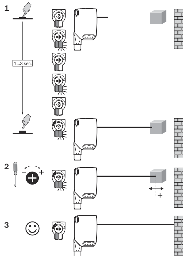
図 68: WTB26x-xxxxxx2xAxx、プッシュターン要素による検出距離の設定
