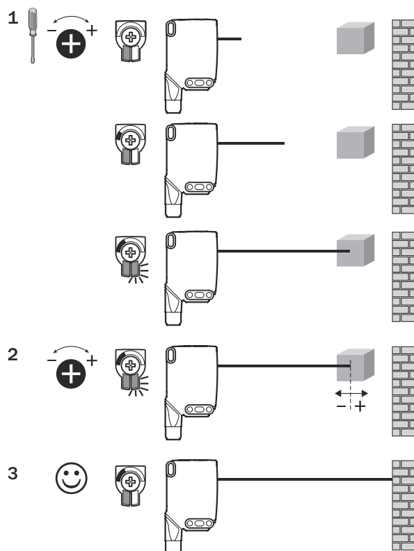
Figura 93: WTB26x-xxxxx1xAxx, ajuste da distância de comutação com potenciômetro
