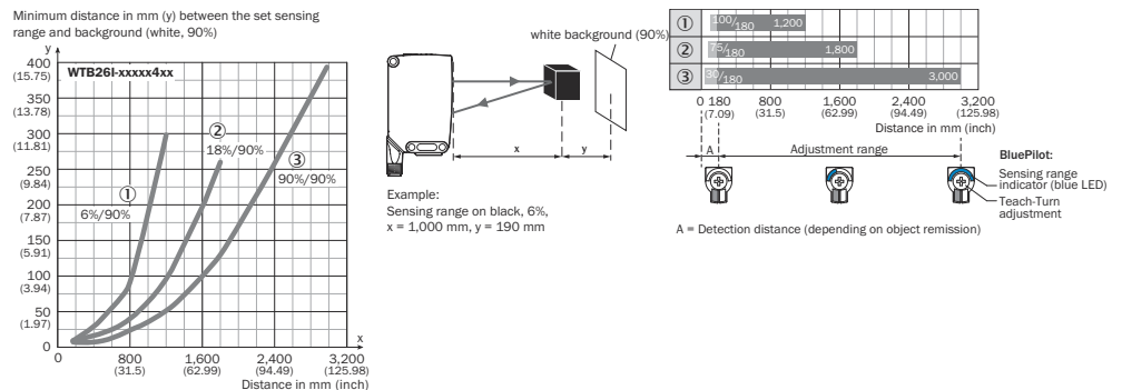
Figura 91: Curva característica 4, WTB26I-xxxxx4xx, luz infravermelha
