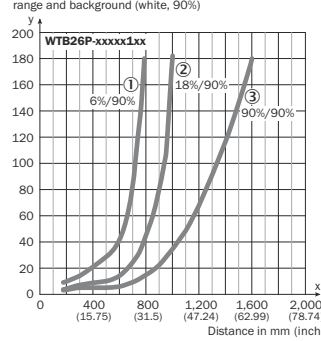
Рисунок 100: Характеристика 1, WTB26P-xxxxx1xx, красный свет
