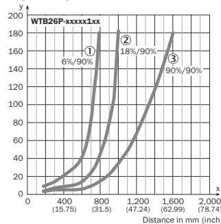
Figura 88: Curva característica 1, WTB26P-xxxxx1xx, luz vermelha
