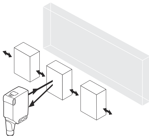
Rysunek 73: Ustawienie czujnika względem kierunku obiektu
