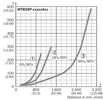
Rysunek 77: Charakterystyka 2, WTB26P-xxxx4xx, światło czerwone
