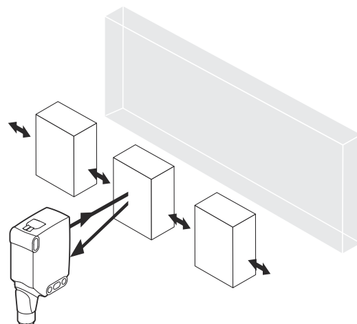
Illustration 37: Alignement du capteur par rapport à la direction de l'objet
