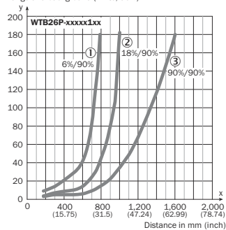
Illustration 40: Caractéristique 1, WTB26P-xxxx1xx, lumière rouge
