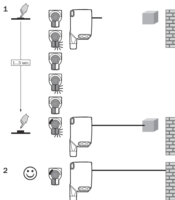
Figura 94: WTB26x-xxxxx3xAxx, ajuste da distância de comutação com tecla teach-in
