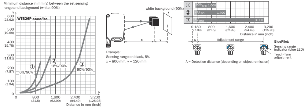
Figura 89: Curva característica 2, WTB26P-xxxxx4xx, luz vermelha
