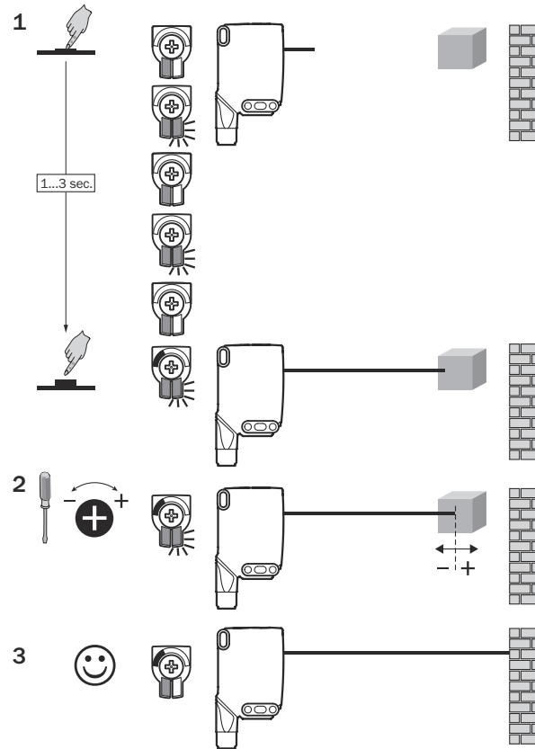
插图 116: WTB26x-xxxxxx2xAxx, 通过按转元件调整触发感应距离
