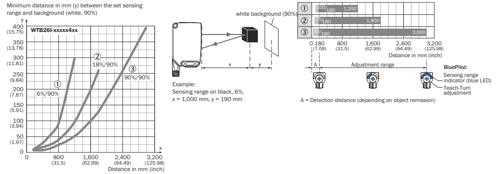
Rysunek 79: Charakterystyka 4, WTB26I-xxxxx4xx, światło podczerwone
