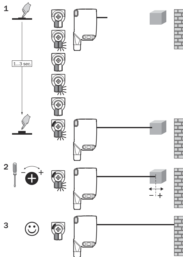
Illustration 44: WTB26-xxxxx2xAxx, réglage de la distance de commutation avec le bouton combiné pousser ou tourner
