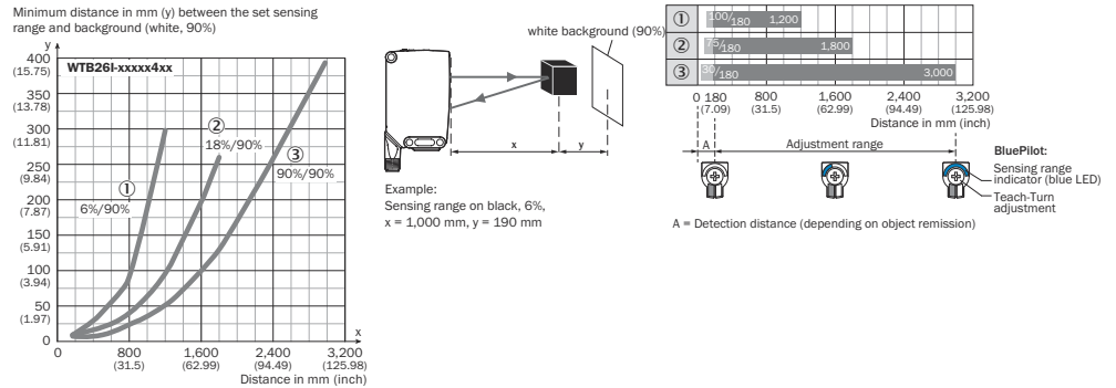
Figura 31: Curva característica 4, WTB26I-xxxxx4xx, luz infrarroja
