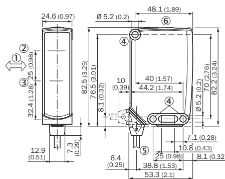
Illustration 47: Plan coté 1, câble
