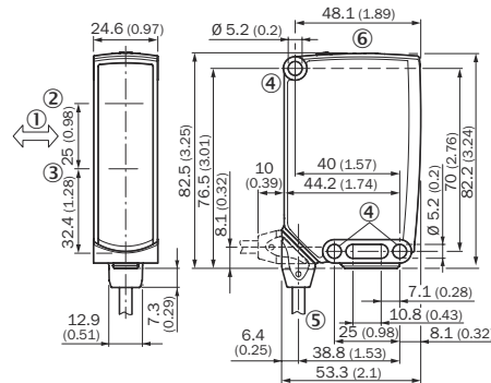
Figura 35: Dibujo acotado 1, cable
