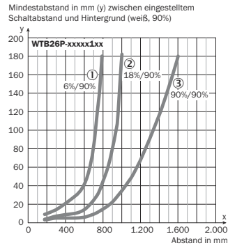
Abbildung 4: Kennlinie 1, WT26P-xxxx1xx, Rotlicht
