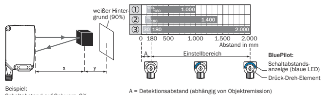
Abbildung 5: Kennlinie 2, WT26P-xxxx4xx, Rotlicht
