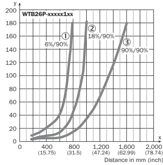
Rysunek 76: Charakterystyka 1, WTB26P-xxxx1xx, światło czerwone
