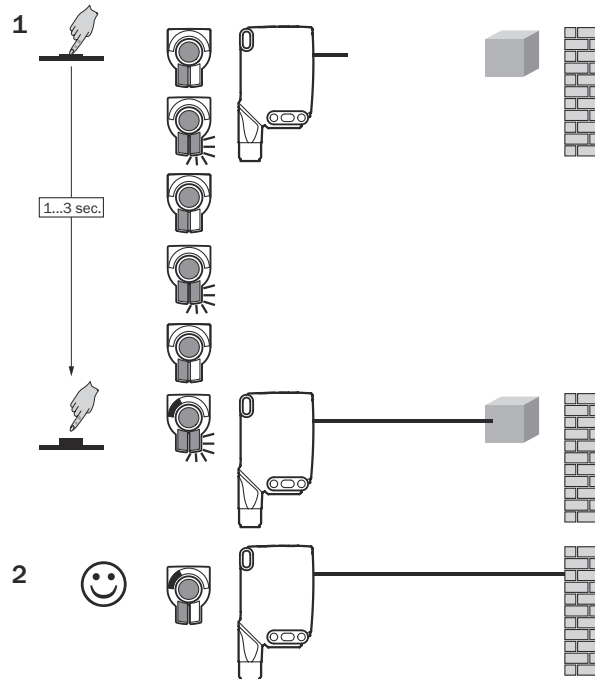
Rysunek 82: WTB26x-xxxxxx3xAxx, ustawianie zasięgu za pomocą przycisku Teach-in
