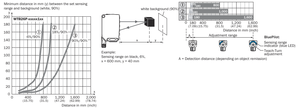
插图 112: 特征曲线 1, WTB26P-xxxx1xx, 红光
