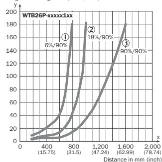
図 64: 特性曲線 1、WTB26P-xxxxx1xx、赤色光
