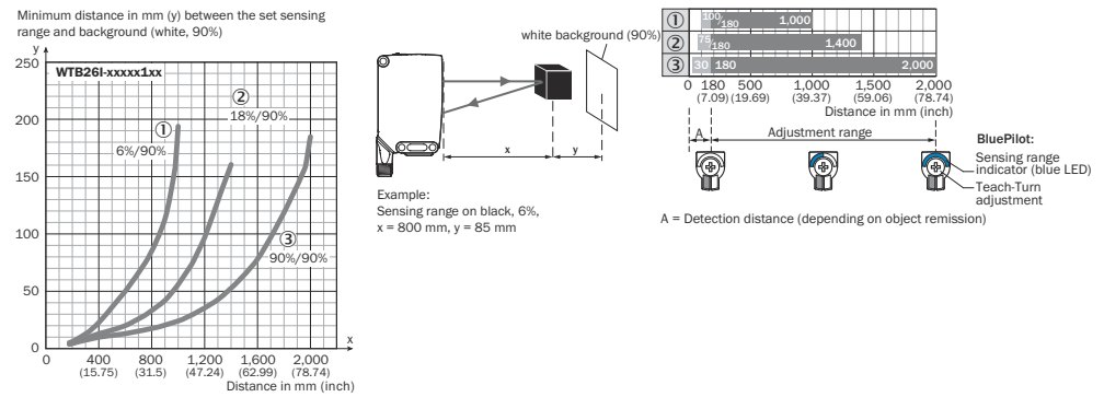
插图 114: 特征曲线 3, WTB26l-xxxxx1xx, 红外光
