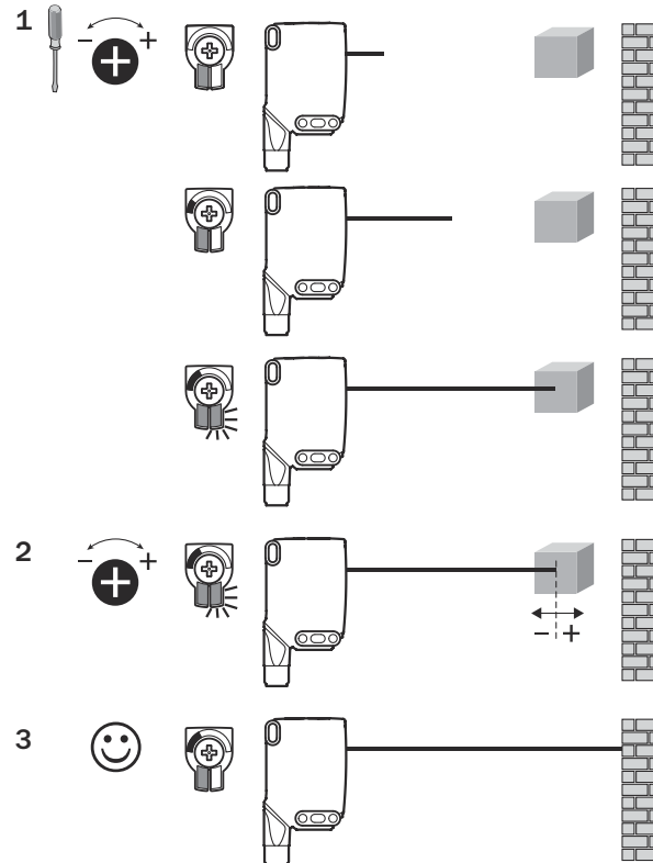
Abbildung 9: WTB26x-xxxxxx1xAxx, Einstellung des Schaltabstands mit Potentiometer
