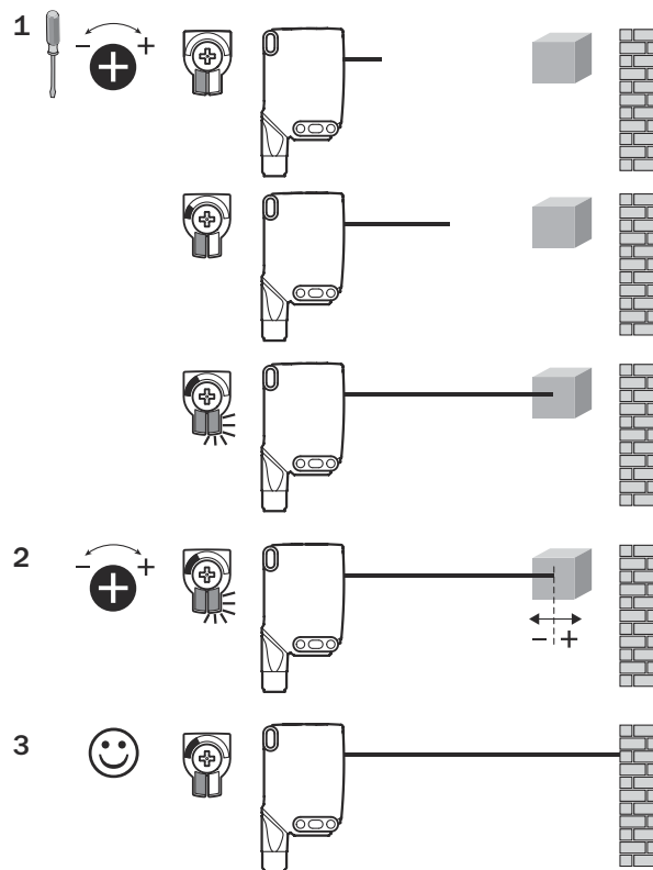
Figura 57: WTB26x-xxxxx1xAxx, impostazione della distanza di lavoro con potenziometro
