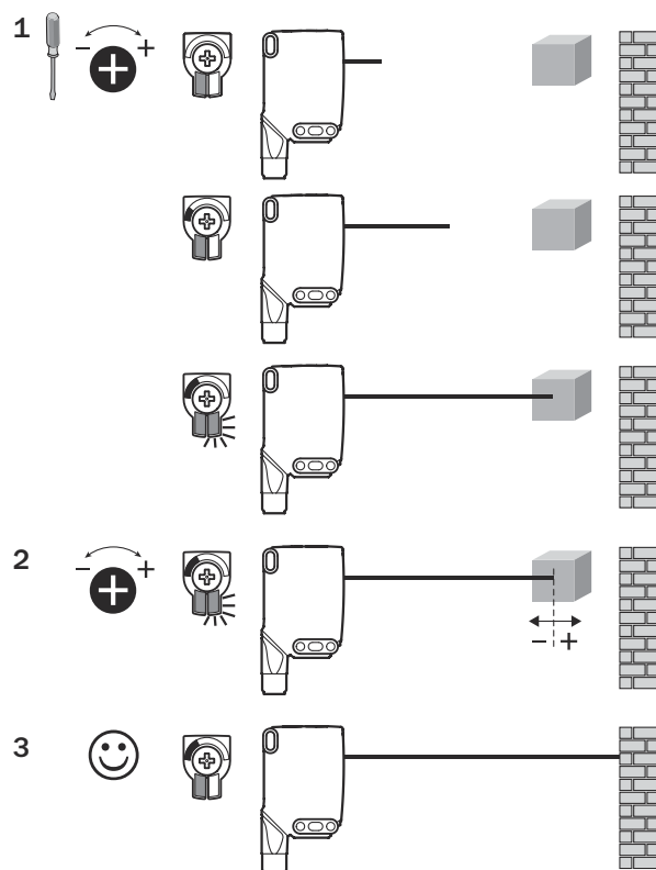
図 69: WTB26x-xxxxxx1xAxx, ポテンシオメータによる検出距離の設定
