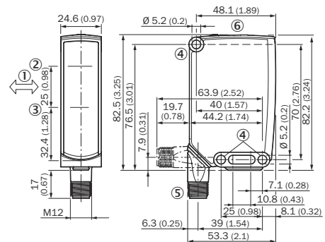
Rysunek 84: Rysunek wymiarowy 2, wtyk
