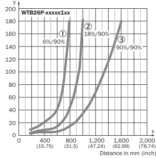
Figura 28: Curva característica 1, WTB26P-xxxx1xx, luz roja
