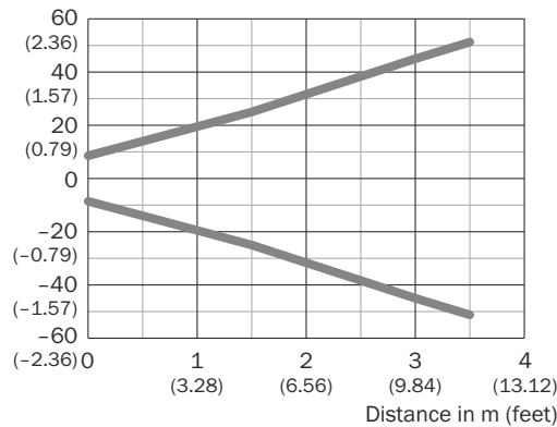
Illustration 20: Taille du spot lumineux, lumière infra rouge
