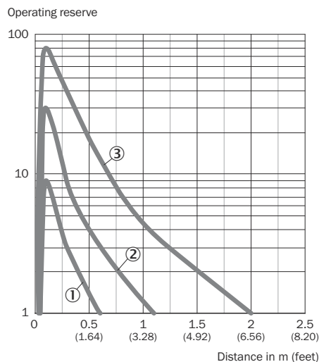
插图 5: 特性曲线, GTE20G, 红光
