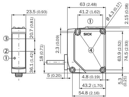
Rysunek 15: GTE20, komora złącza zaciskowego
