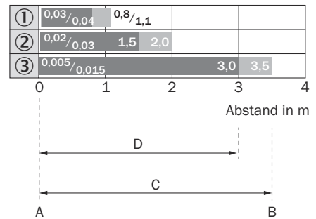
Abbildung 8: Schaltabstandsdiagramm, GTE20M, Infrarotlicht
