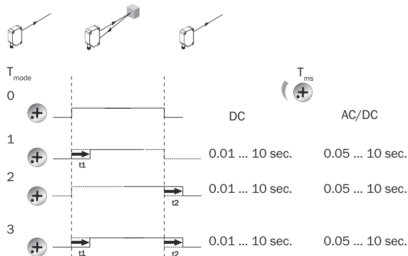
Figura 11: Funzioni temporali
