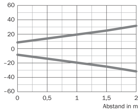
Abbildung 19: Lichtfleckgröße, rotes Licht
