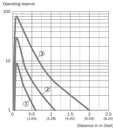
図 5: 特性曲線、GTE20G、赤色光
