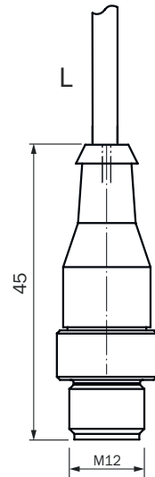
Illustration 16: Connecteur M12
