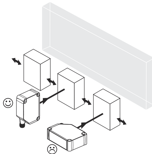
Abbildung 3: Ausrichtung des Sensors relativ zur Objekttrichtung
