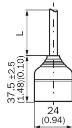
Figura 18: Connettore Q7
