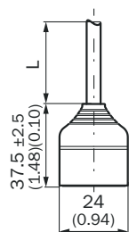
図 18: コネクタ Q7
