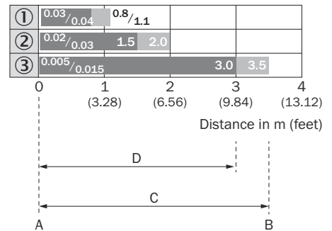
Rysunek 8: Wykres zasięgu, GTE20M, światło podczerwone
