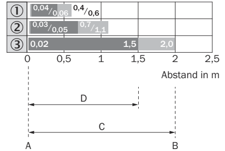
Abbildung 6: Schaltabstandsdiagramm, GTE20G, Rotlicht
