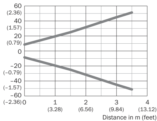
插图 20: 光点尺寸, 红外线
