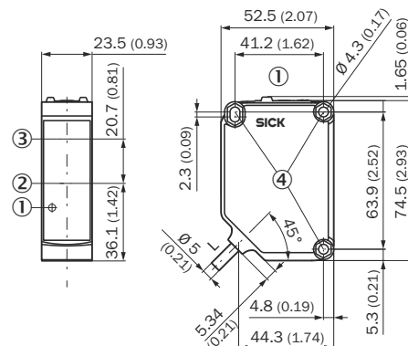
図 14: GTE20, ケーブル
