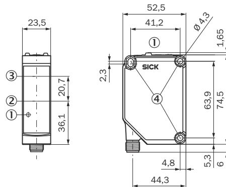
Abbildung 13: GTE20, M12-Steckverbinder
