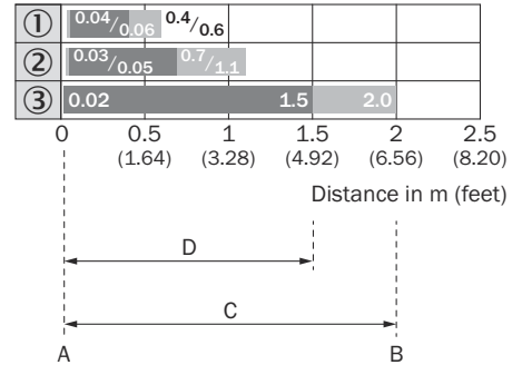
Illustration 6: Diagramme de distance de commutation, GTE20G, lumière rouge
