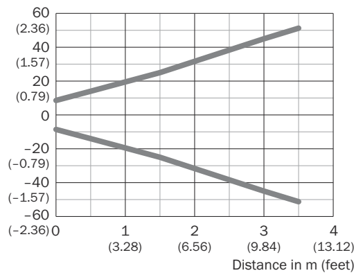
Figura 20: Tamanho do ponto de luz, luz infravermelha
