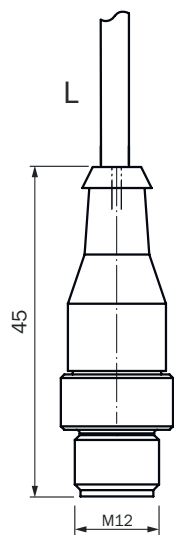
插图 16: 连接器 M12
