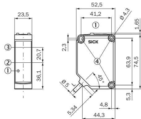
Abbildung 14: GTE20, Leitung
