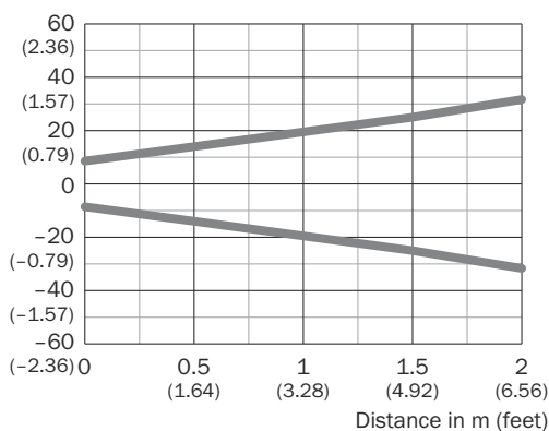
図 19: レーザスポットサイズ、赤色光
