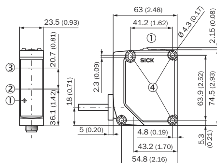
図 15: GTE20, 端子チャンバ
