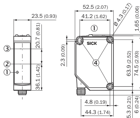
図 13: GTE20, M12 コネクタ
