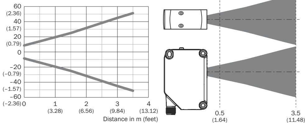
図 20: レーザスポットサイズ、赤外光
