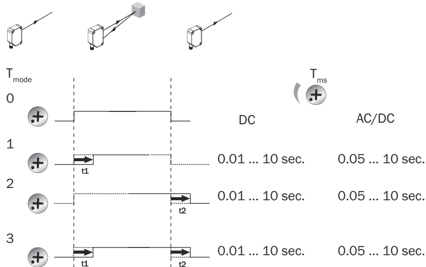
Illustration 11: Fonctions temporelles
