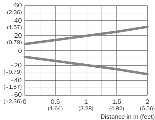
Figura 19: Tamanho do ponto de luz, luz vermelha
