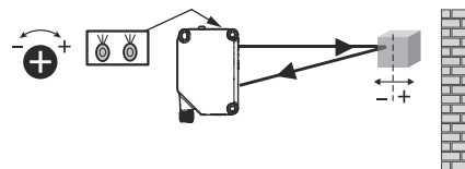
図 9: 調整
