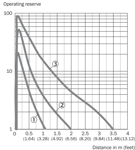
図 7: 特性曲線、GTE20M、赤外光
