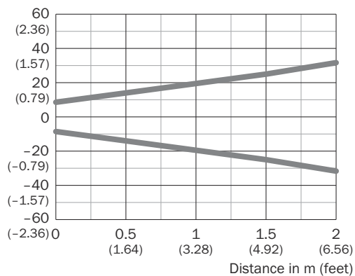
插图 19: 光点尺寸, 红光
