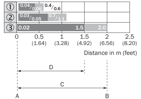
Figura 6: Digramma della distanza di lavoro, GTE20G, luce rossa
