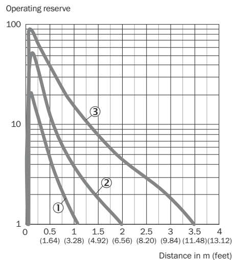
Illustration 7: Ligne caractéristique, GTE20M, lumière infra rouge
