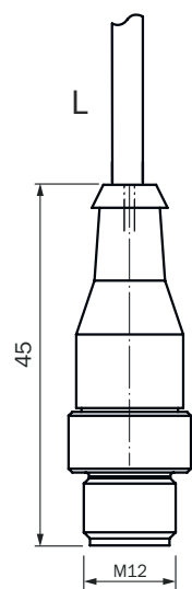
図 16: コネクタ M12
