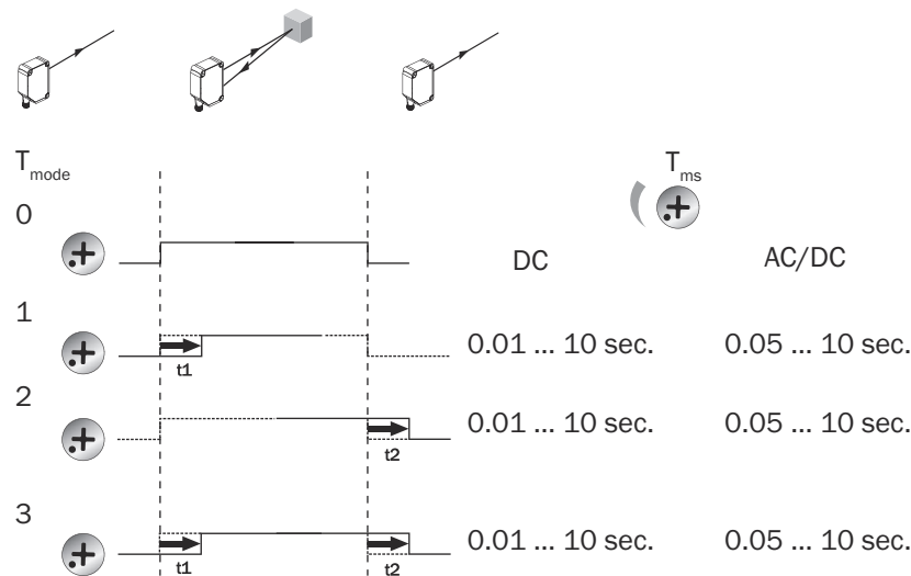
図 11: タイマー機能
