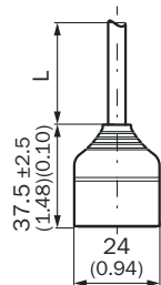
插图 18: 连接器 Q7
