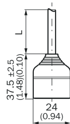
Rysunek 18: Złącze Q7
