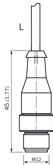
Abbildung 16: M12-Steckverbinder
