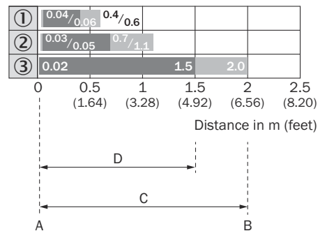
Figura 6: Diagrama da distância de comutação, GTE20G, luz vermelha
