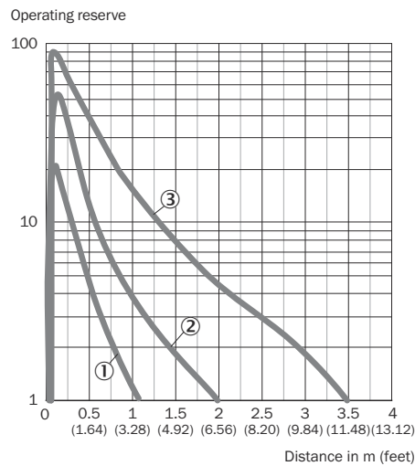
Figura 7: Curva característica, GTE20M, luz infrarroja
