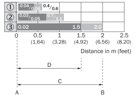
図 6: 検出距離図、GTE20G、赤色光
