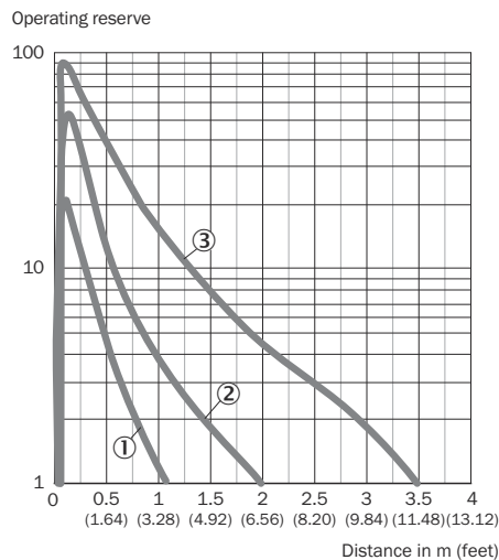
Figura 7: Curva característica, GTE20M, luz infravermelha
