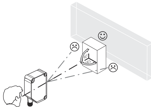
Figura 4: Allineamento 1
