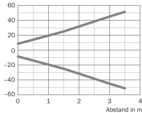
Abbildung 20: Lichtfleckgröße, Infrarotlicht
