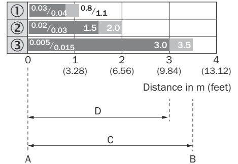
図 8: 検出距離図、GTE20M、赤外光
