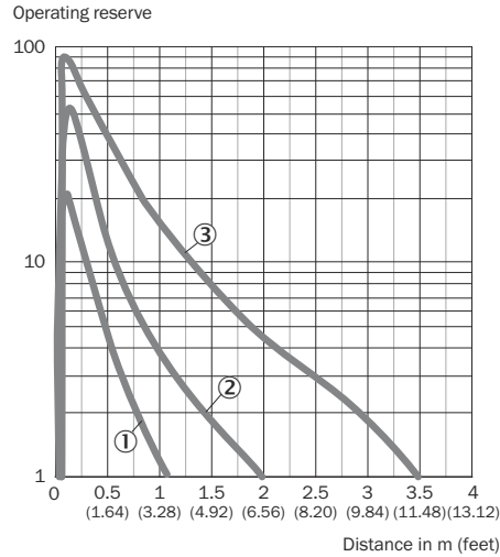
插图 7: 特性曲线, GTE20M, 红外线
