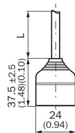
Illustration 18: Connecteur Q7
