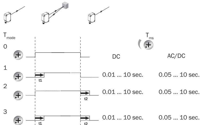
Figura 11: Funções de tempo
