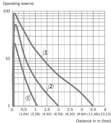
Figura 7: Curva caratteristica, GTE20M, luce infrarossa
