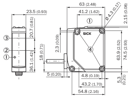
Illustration 15: GTE20, boîte de raccordement
