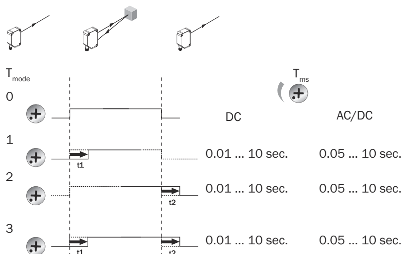
插图 11: 时间功能
