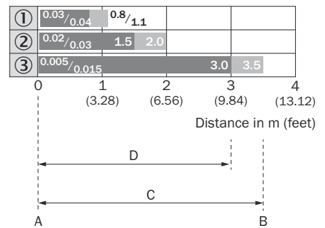
Illustration 8: Diagramme de distance de commutation, GTE20M, lumière infra rouge
