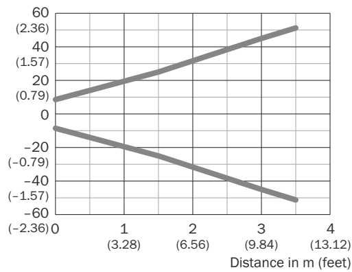
Figura 20: Dimensioni punto luminoso, luce infrarossa
