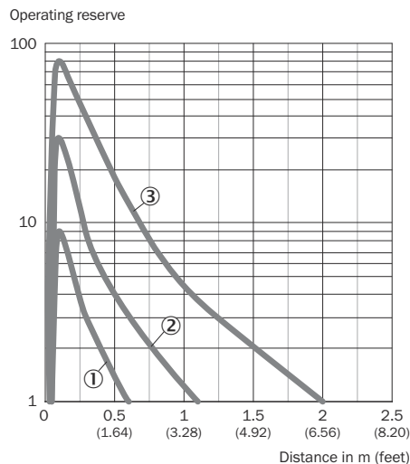
Figura 5: Curva característica, GTE20G, luz vermelha
