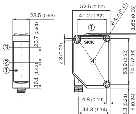
插图 13: GTE20, M12 连接器
