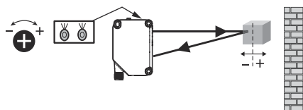
Figura 9: Ajuste
