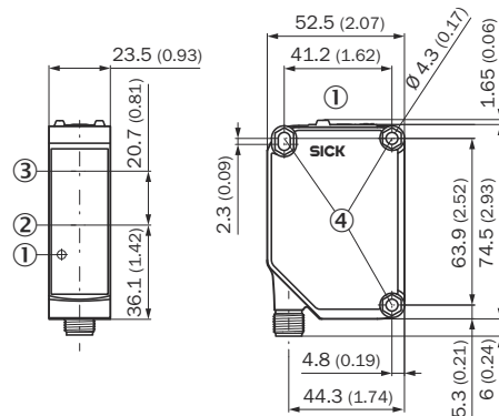
Figura 13: GTE20, conector M12
