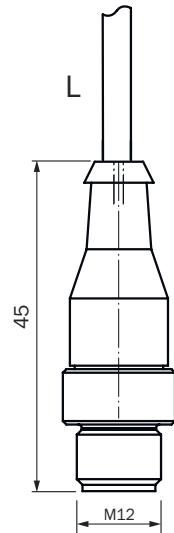
Rysunek 16: Złącze M12
