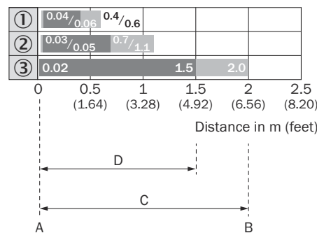
插图 6: 触发感应距离图表, GTE20G, 红光
