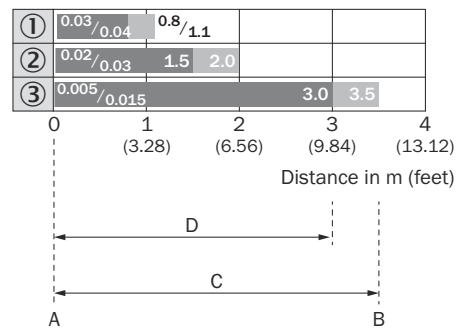
Figura 8: Diagrama da distância de comutação, GTE20M, luz infravermelha
