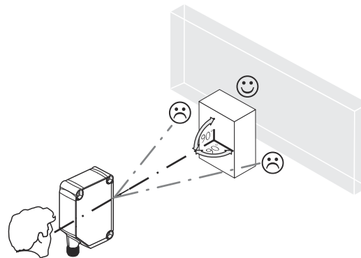
Abbildung 4: Ausrichtung 1
