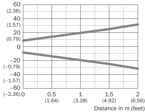
Figura 19: Tamaño del spot, luz roja
