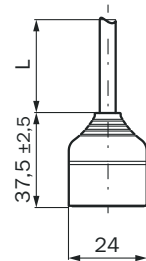
Abbildung 18: Q7-Steckverbinder
