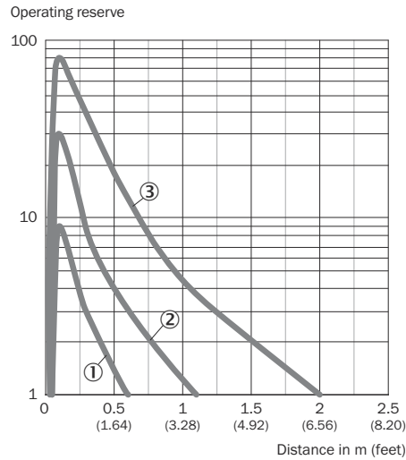
Rysunek 5: Krzywa charakterystyki, GTE20G, światło czerwone
