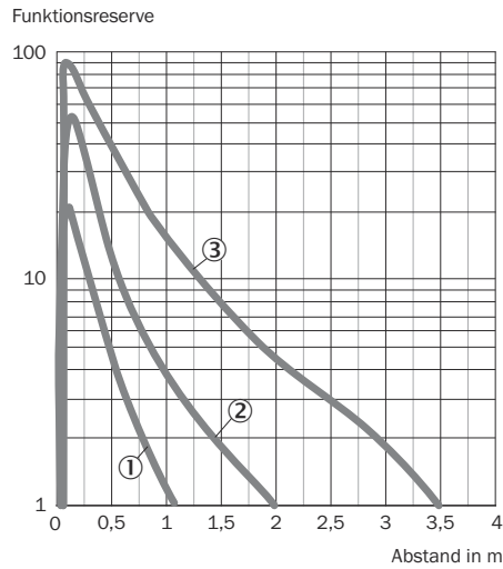
Abbildung 7: Kennlinie, GTE20M, Infrarotlicht
