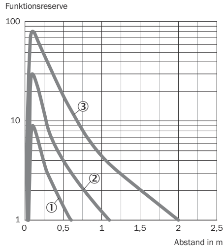
Abbildung 5: Kennlinie, GTE20G, Rotlicht
