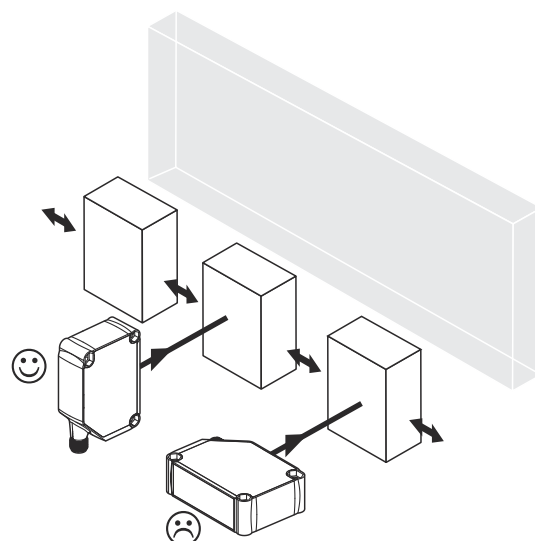
Figura 3: Orientamento del sensore rispetto alla direzione dell'oggetto
