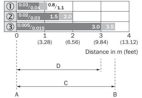
插图 8: 触发感应距离图表, GTE20M, 红外线
