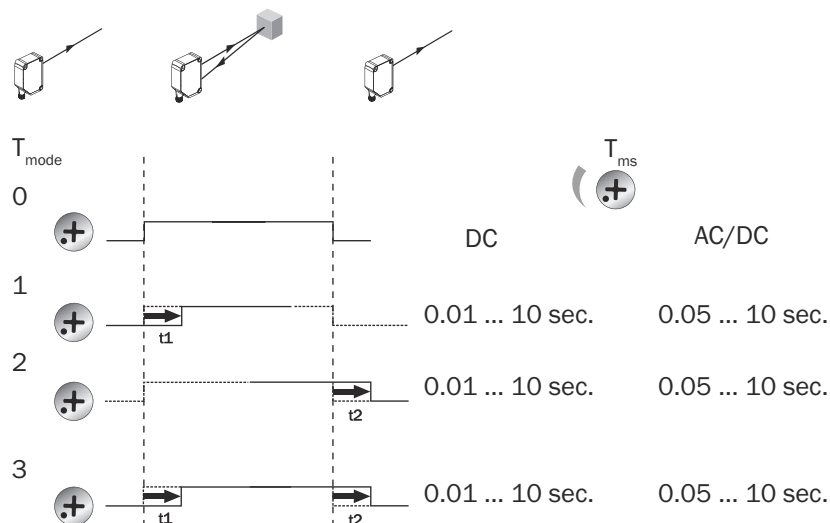
Rysunek 11: Funkcje czasu
