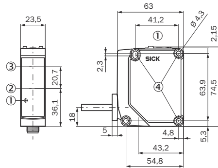
Abbildung 15: GTE20, Anschlussgehäuse
