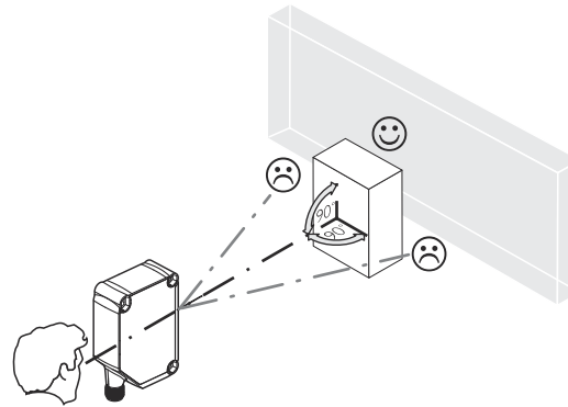
図 4: 光軸調整 1
