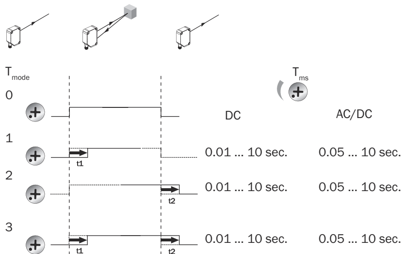
Figura 11: Funciones de temporización
