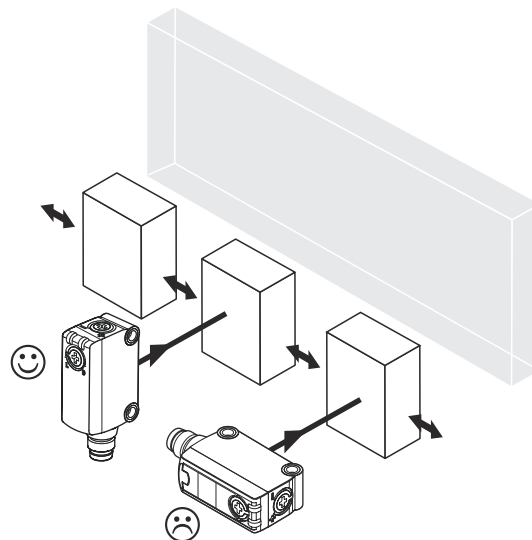
Abbildung 3: Ausrichtung der Lichtschranke relativ zur Objektrichtung
