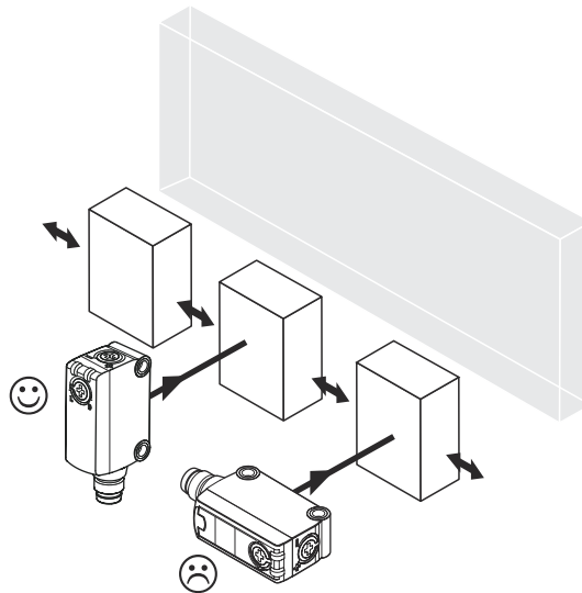
Figura 3: Orientação do sensor em relação à direção do objeto
