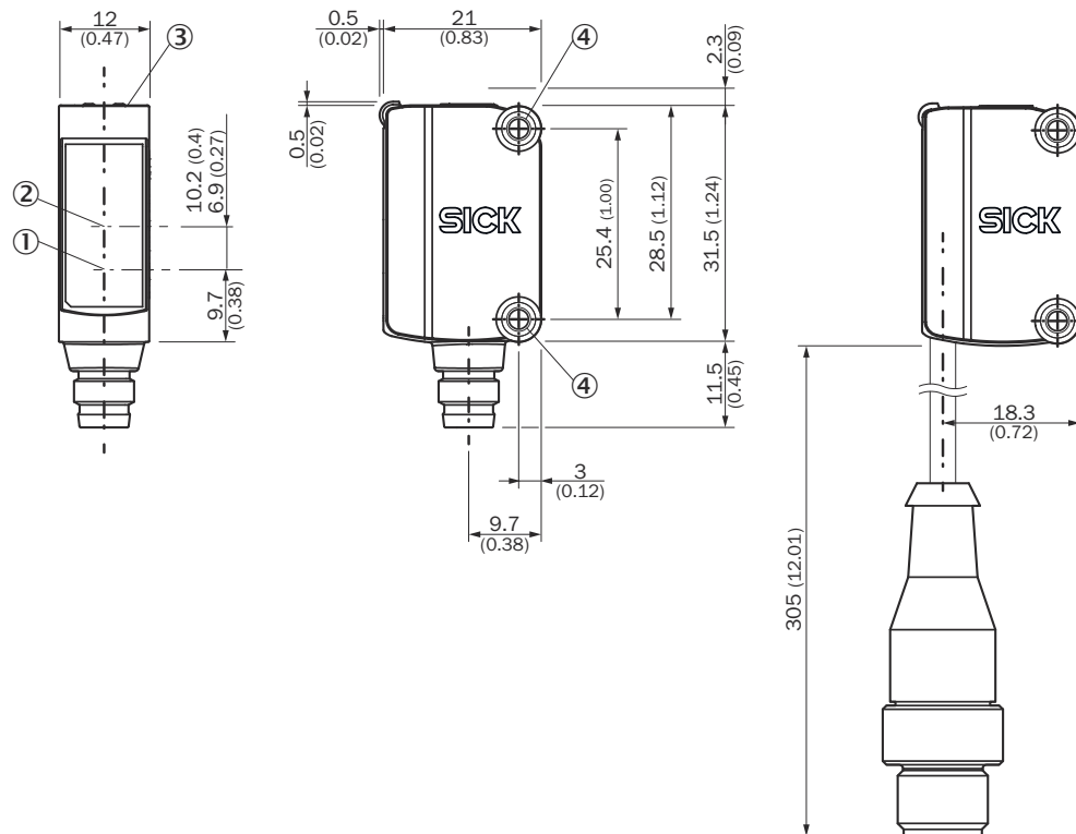
Figura 7: Desenho dimensional
