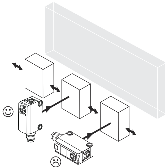
插图 3: 相对于物体方向的传感器取向
