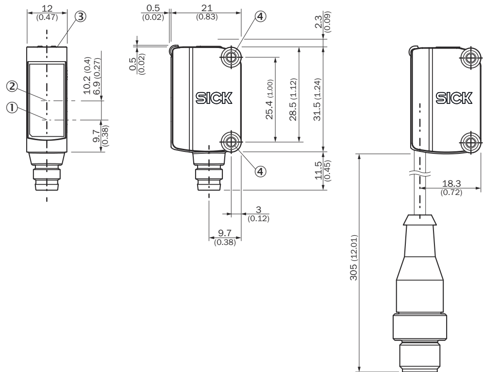
Figura 7: Dibujo acotado
