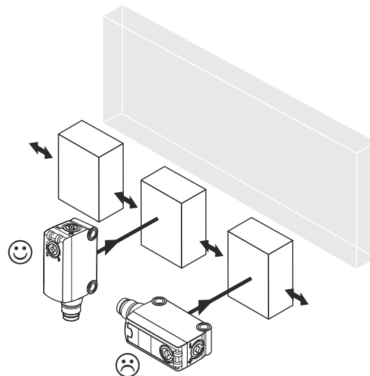
Rysunek 3: Ustawienie czujnika w stosunku do kierunku obiektu
