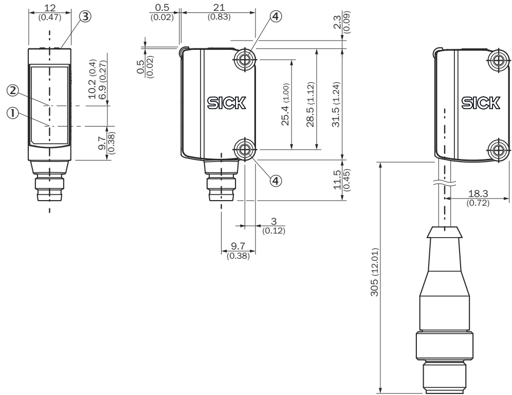
그림 7: 치수 도면
