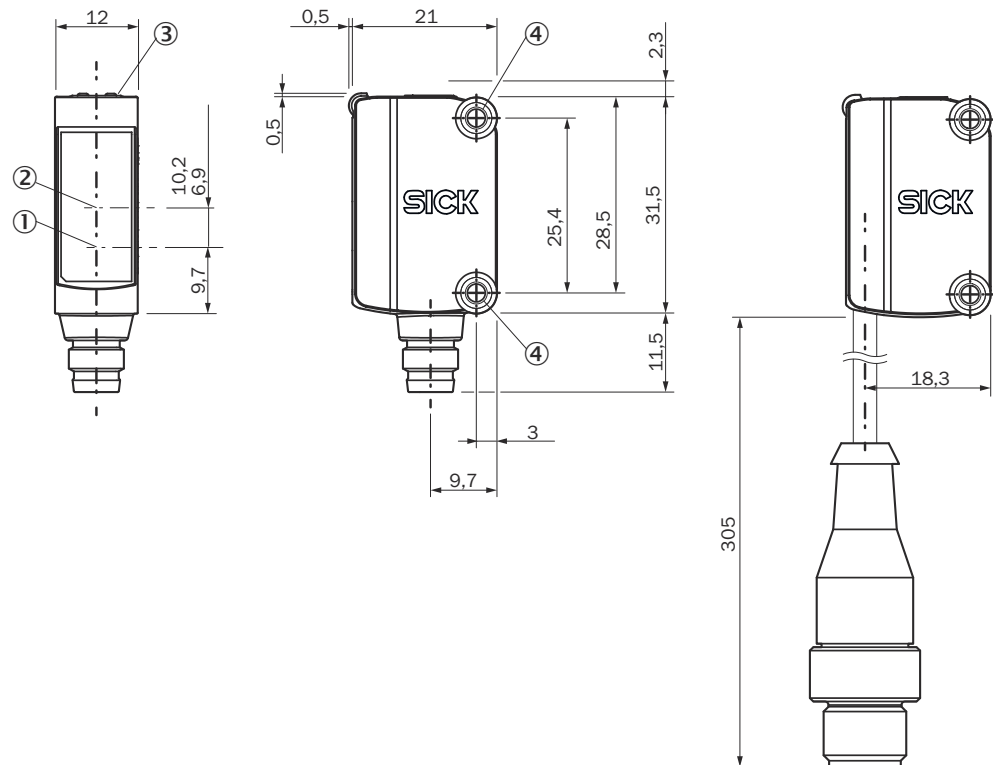
Abbildung 7: Maßzeichnung
