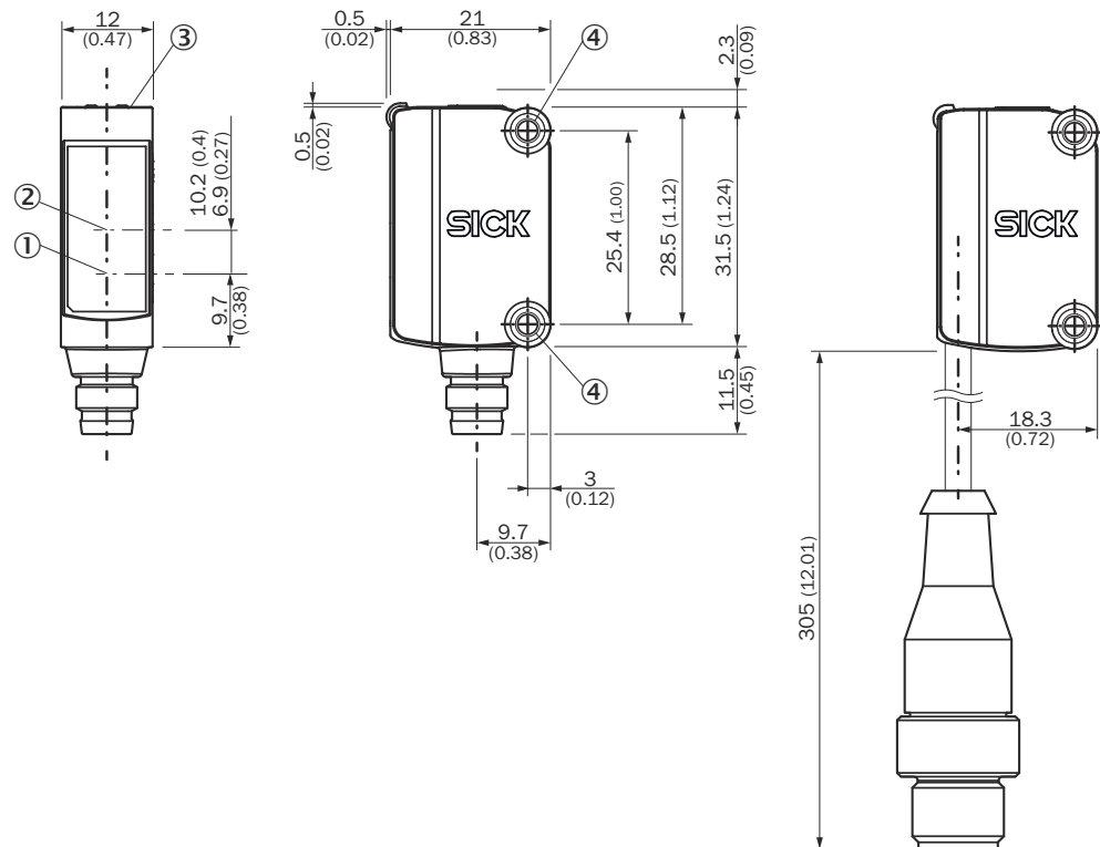
Rysunek 7: Rysunek wymiarowy
