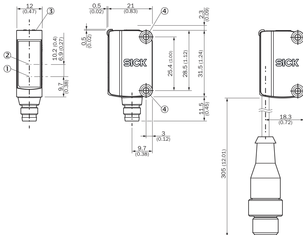
図 7: 寸法図
